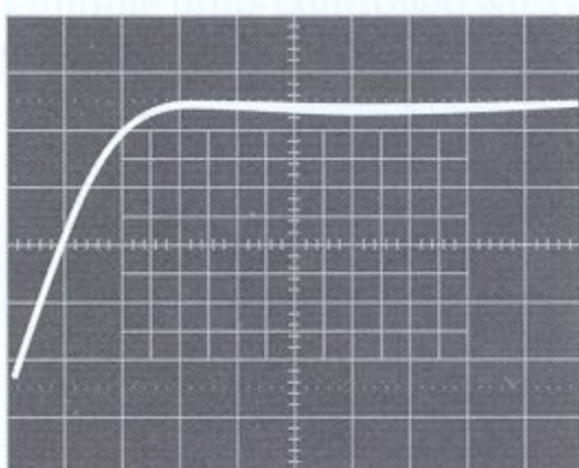
Actual 228A transient response, 100V range @ 1A. Vert.: 20V/div. Horiz.: 0.2ms/div.
